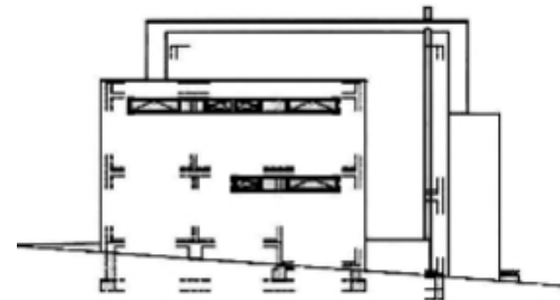
Ansicht Nord.
